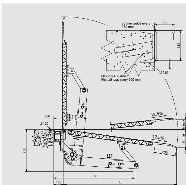
SKB pohyblivý s pružinovým systémem
