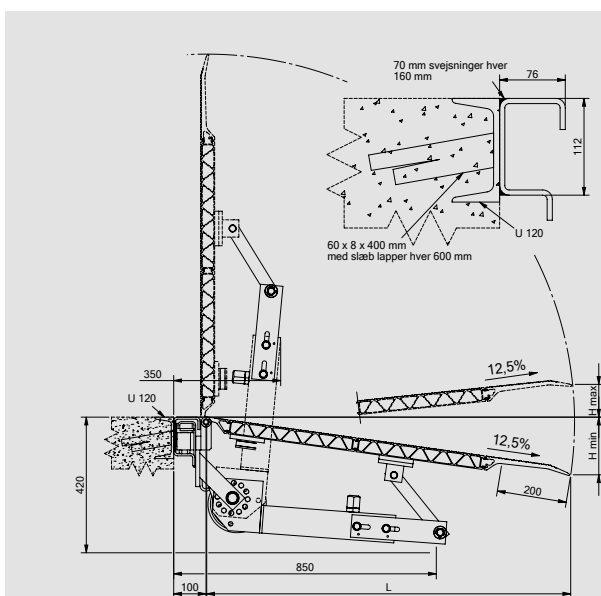
SKB flytbar med fjedersystem
